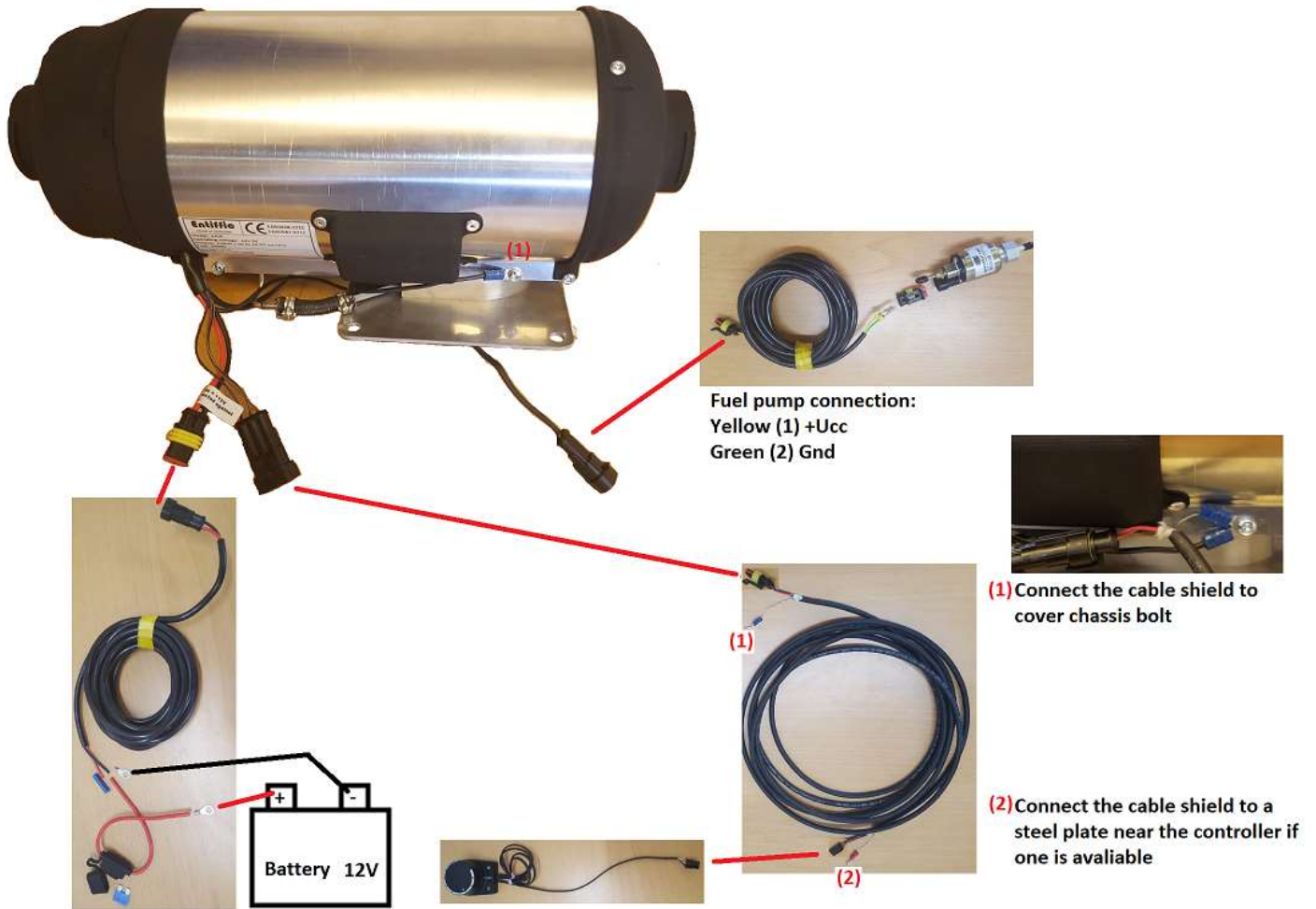
Figur 10 Elektriske forbindelser
